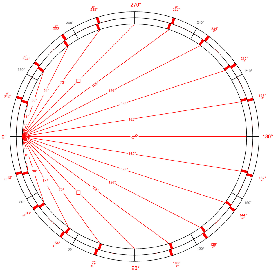
Figure 7 : graphique des aspects de talent. Les orbes de cette série sont de \pm 1^\circ .
