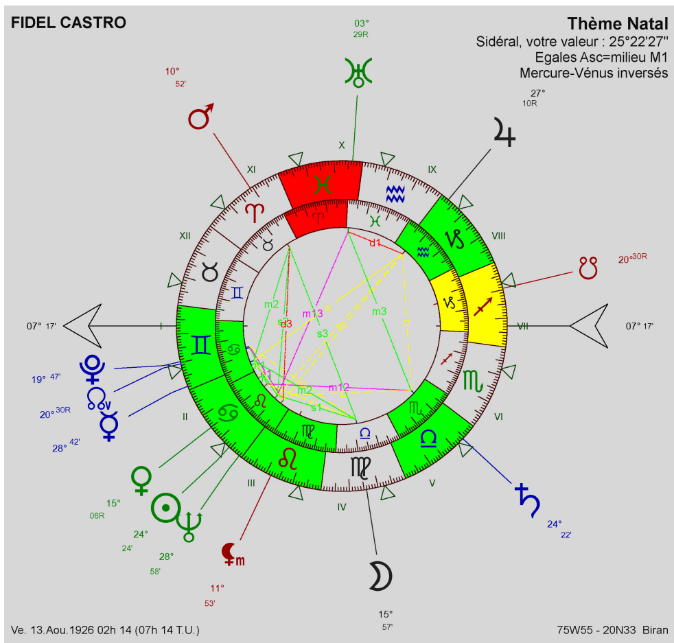
Figure 43 : la carte du ciel de Fidel Castro.
