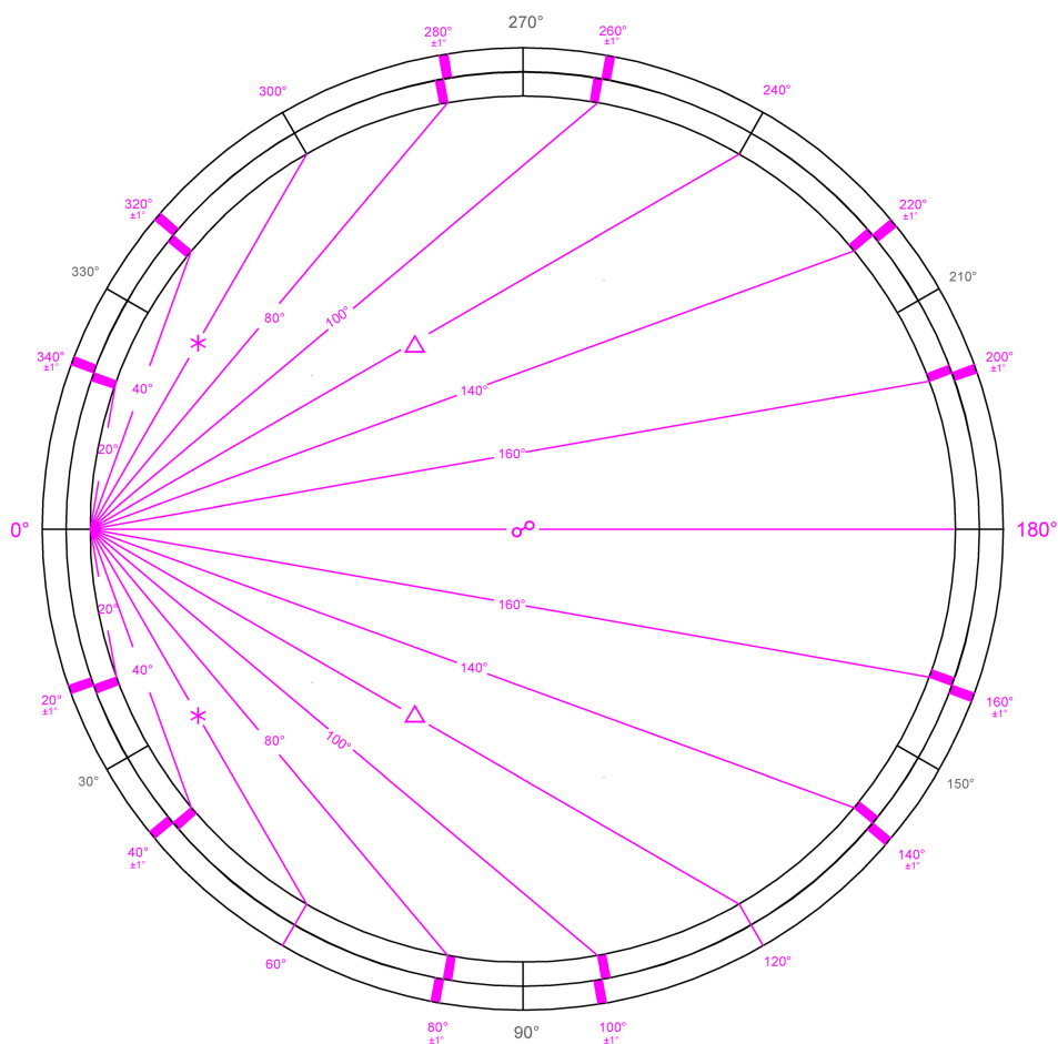
Figure 8 : graphique des aspects de recherche. Les orbis de cette série sont de \pm 1^\circ .
