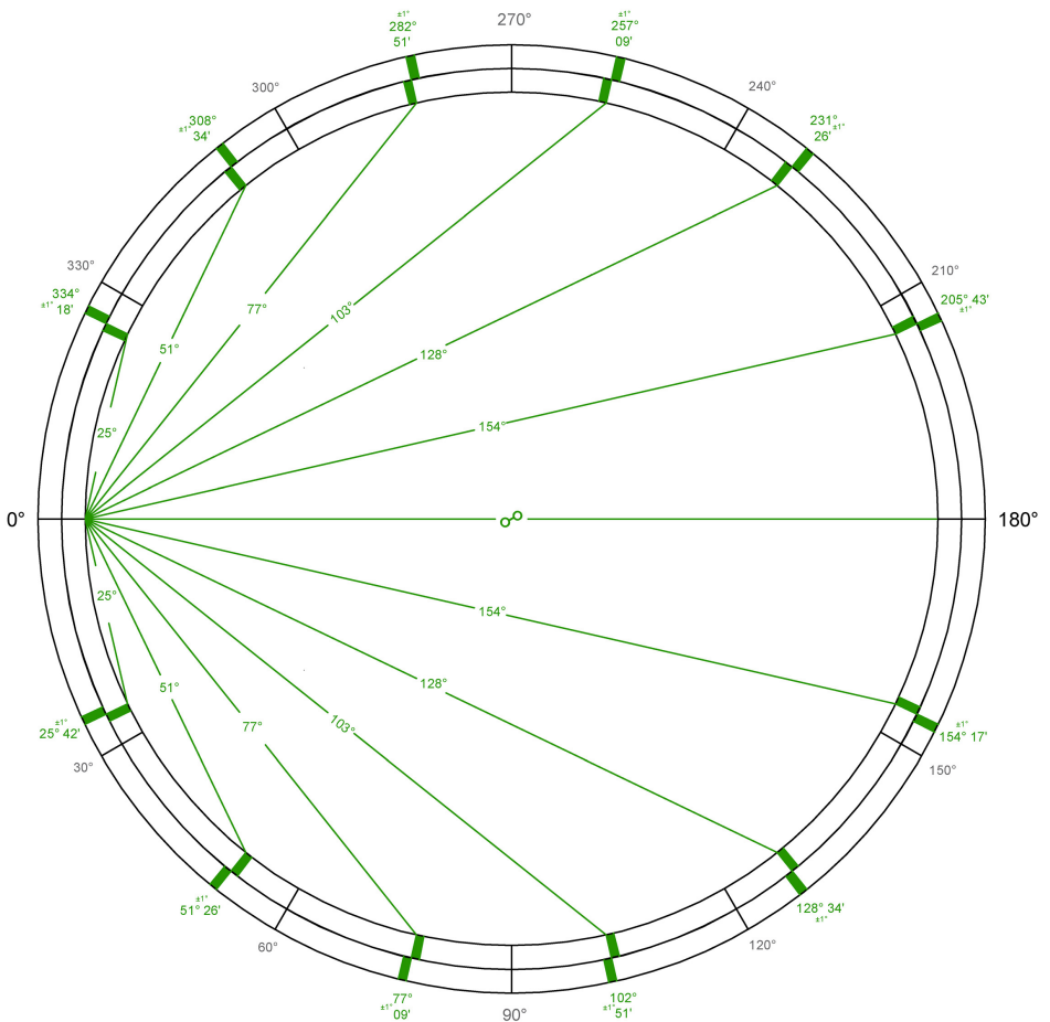
Figure 6 : graphique des aspects de mission. Les orbes de cette série sont de \pm 1^\circ .
