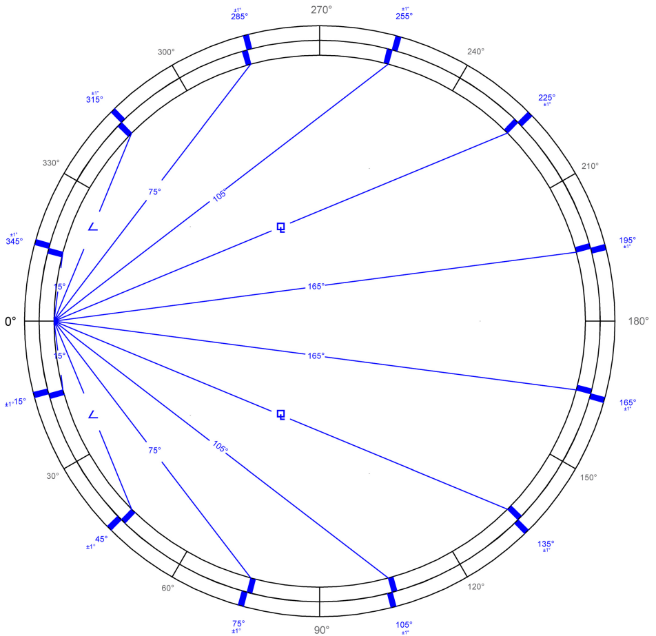
Figure 5 : graphique des aspects de blocage. Les orbales de ces aspects sont de \pm 1^\circ .
