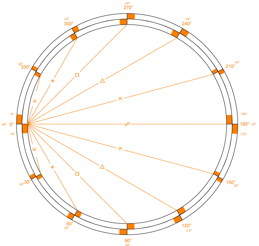
Figure 4 : graphique des aspects énergétiques et de leurs orbes. Ceux-ci ont été colorés en orange plutôt qu'en jaune pour une meilleure visibilité sur le fond blanc.
